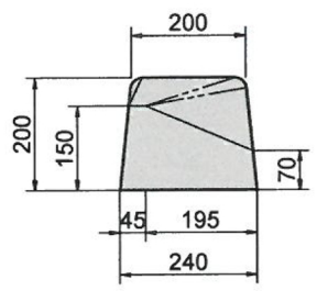
C型据付ブロック 両面 質量 51kg
