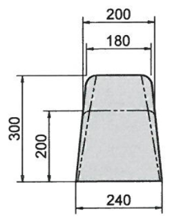
D型据付ブロック 両面 質量 87kg
