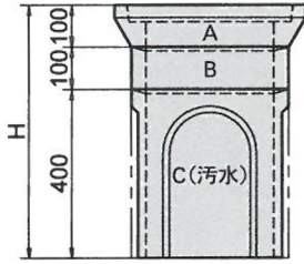
TMS30(SK)汚水
