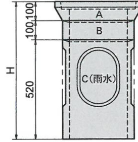
TMR30(RK)雨水
