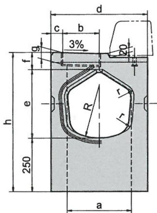
境界ブロック用ます（VM-E型）
