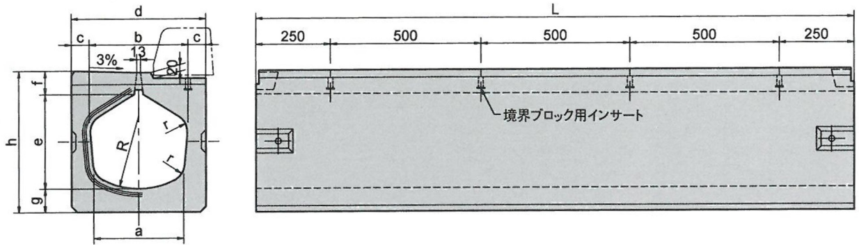
境界ブロック用側溝（V-E型）
