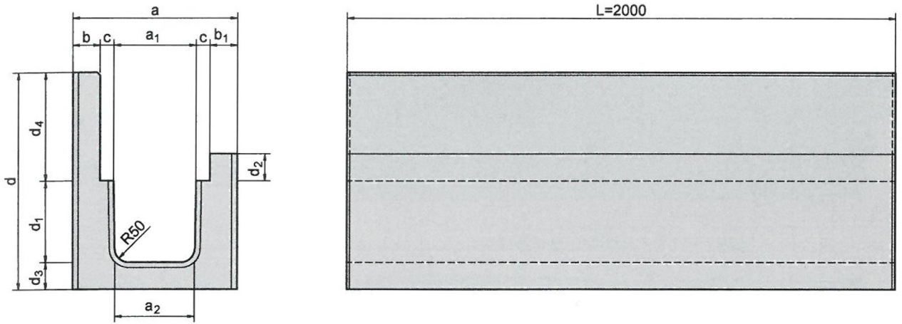
土留め付歩車道用 240 (HC120×120)
