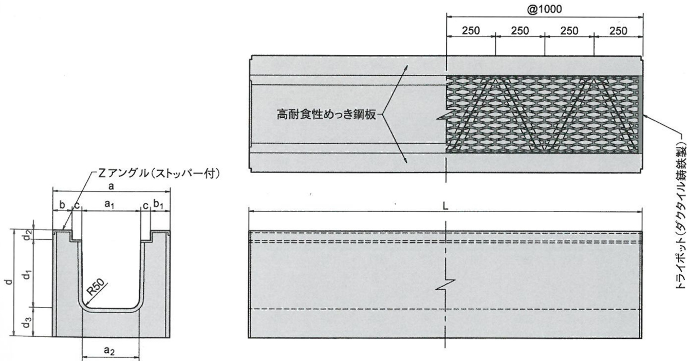
重耐型横断用 (TD150×150)
