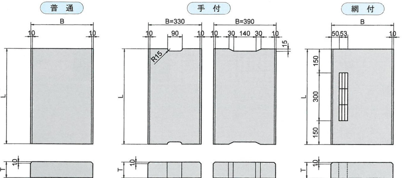
鉄筋コンクリート埼玉県型甲蓋（車道用）
