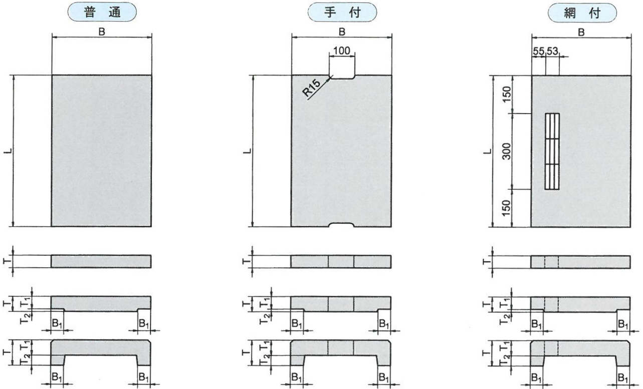
鉄筋コンクリート埼玉県型甲蓋（歩道用）
