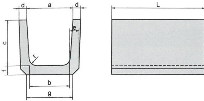
U形側溝 及び 上ぶた式U形側溝（本体）
